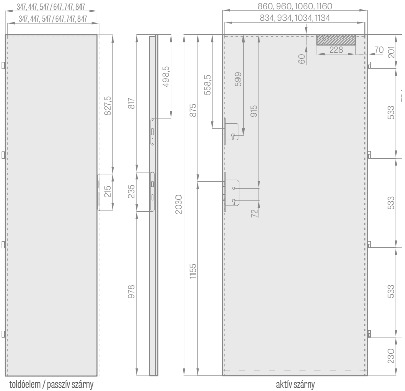
toldóelem / passzív szárny
